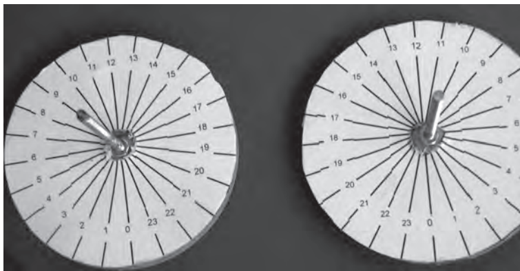
Fig. 6. Cadrans équatoriaux polaires, divisés en 24 secteurs de 15°, gradués en sens inverse (le cadran nord, dans le sens inverse des aiguilles d'une montre ; le cadran du pôle Sud, dans le sens des aiguilles).
