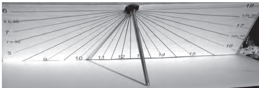
Fig. 8. Étalonage d'un cadran horizontal en un lieu, à partir d'un cadran équatorial de ce lieu.
