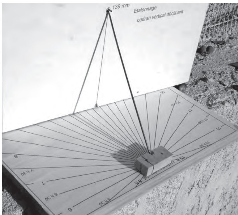
Fig. 9. Étalonage d'un cadran vertical en un lieu, à partir d'un cadran horizontal de ce lieu.
