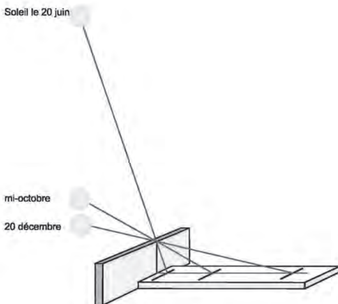
Fig. 2. Maquette du cadran solaire égyptien du temps de Thutmosis III (xv e siècle av. J.-C.) qui passe pour le plus ancien cadran connu.
