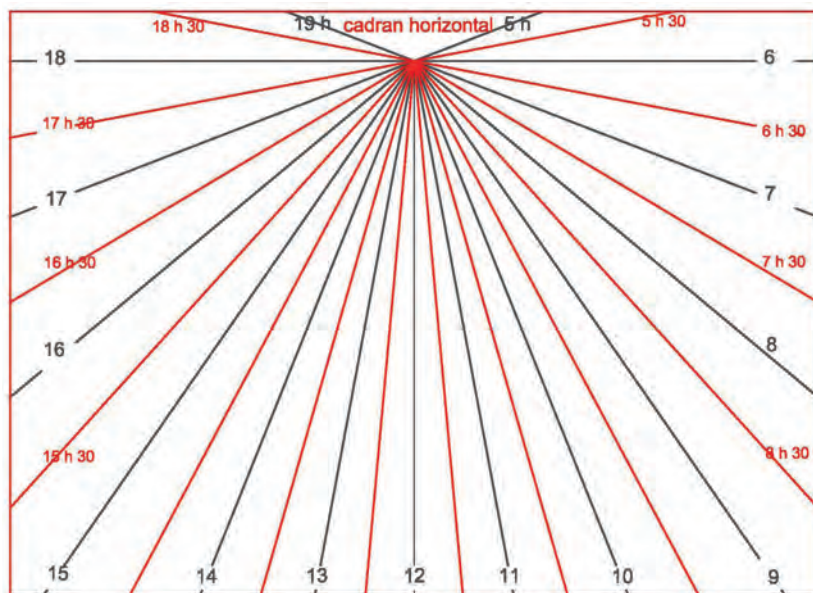
Fig. 7. Cadran solaire équatorial en un lieu. Il s'obtient simplement en transportant les cadrans solaires polaires parallèlement à eux-mêmes.
