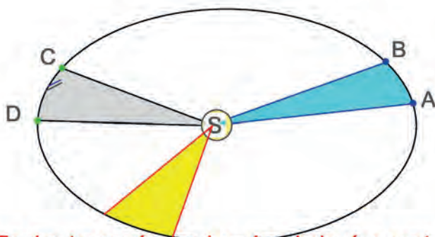
Fig. 12. La loi des aires selon laquelle le rayon soleil-terre parcourt en des temps égaux des aires égales. Il s'ensuit des inégalités dans la durée des jours solaires, ce qui se traduira par des corrections nécessaires à apporter pour passer des jours solaires indiqués par les cadrans et notre montre.
