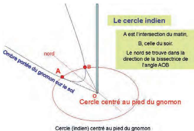
Fig. 5. Les cercles indiens, centrés au pied du gnomon, permettent de déterminer la direction du nord, de s'orienter et de fixer le méridien d'un lieu.
