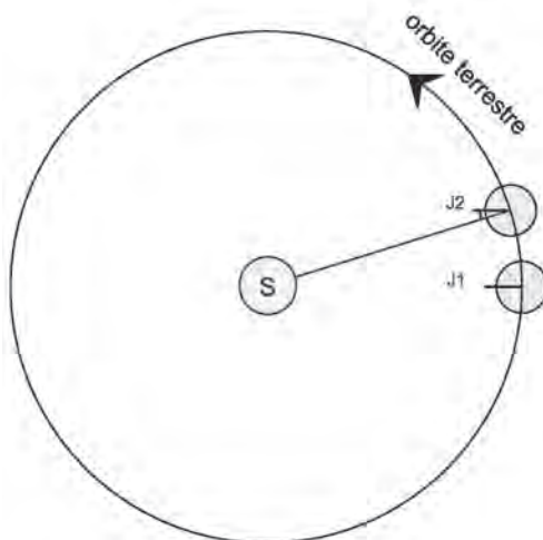
Fig. 11. Jour solaire et jour sidéral.
