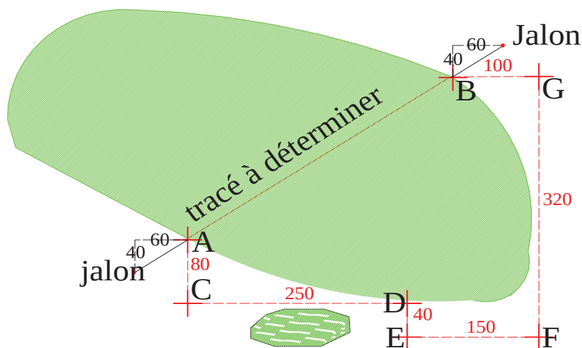
Fig. 7. Sur le terrain, pour relier deux points non visibles l'un de l'autre, on peut décomposer le parcours global en une suite de parcours élémentaires, rectilignes, dirigés selon les directions principales, nord-sud ou est-ouest.
