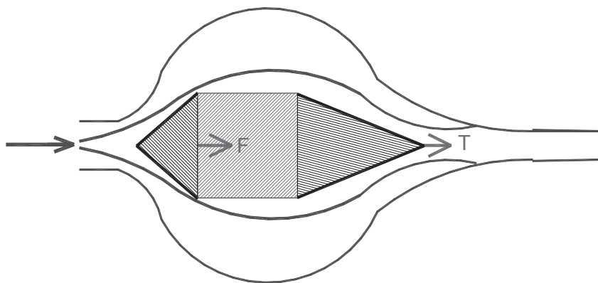
Fig. 5. Avant-bec et arrière-bec protègent les deux faces de la pile. L'arrière-bec réduit les forces de suction.
