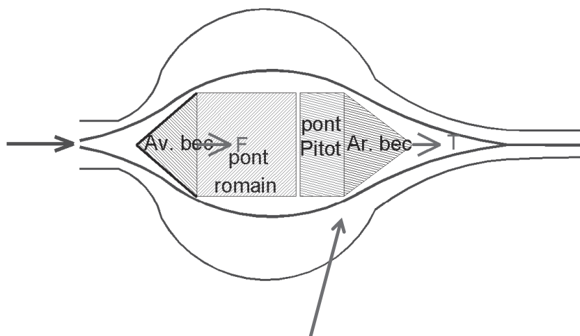
Fig. 6. Au pont du Gard, le pont routier n'étant pas solidaire du pont romain, la force de succion « T » n'exerce aucune action sur ce dernier.
