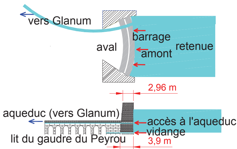
Fig. 2. Le barrage-voûte du Peyrou (aqueduc de Glanum).
