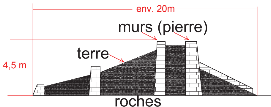
Fig. 1. Barrage-masse de Jerwan (IV e millénaire).
