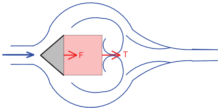
Fig. 4. L'avant-bec protège la pile, en amont, des courants incidents.
